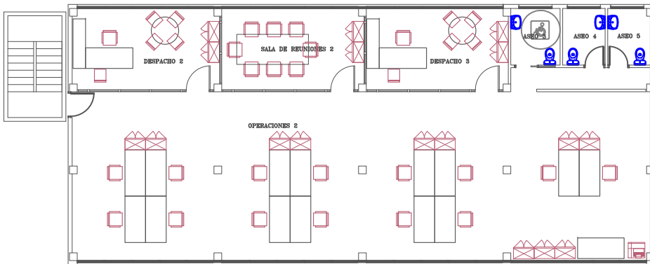
PLANTA PRIMERA
