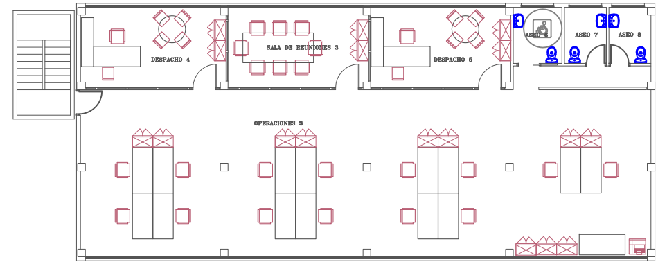
PLANTA SEGUNDA
