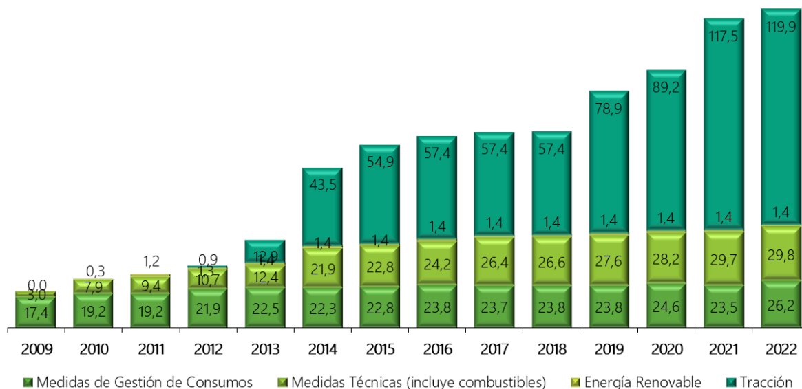
Gráfica 7. Realizaciones a 31 de diciembre de cada año de los Planes de Implantación de Acciones de Ahorro y Eficacia Energética y Sistemas de Generación de Energía Renovable en Adif y Adif-Alta Velocidad (Ahorros conseguidos en GWh/año)
