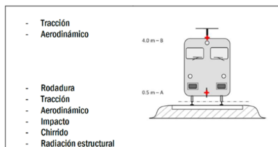
Figura 18. Fenómenos que contribuyen a la emisión.
